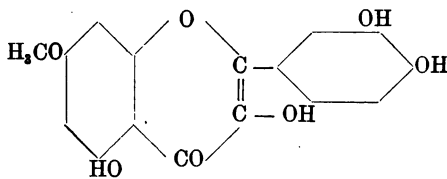
Rhamnetin.
